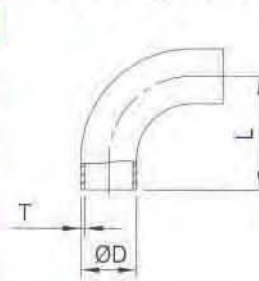
90° Long Bend C.L2S-90° Bend
